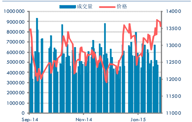
沪胶成交量
