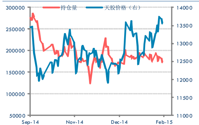
沪胶持仓量
